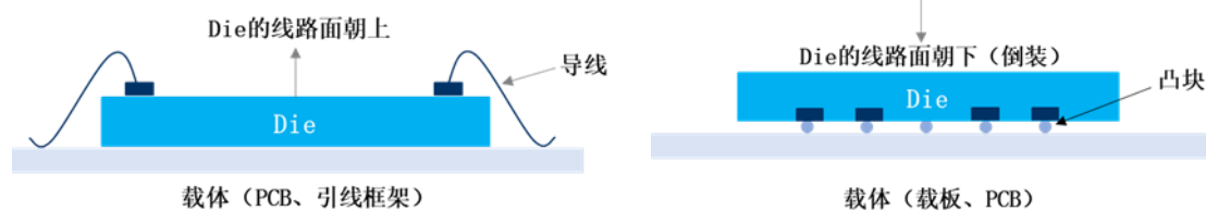
传统封装（打线）与先进封装（倒装）对比
