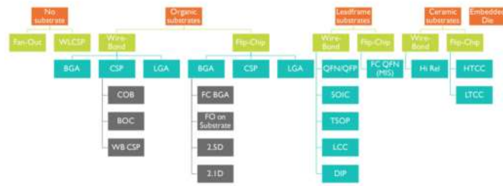
集成电路封装形式的分类
